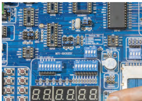
开发板
